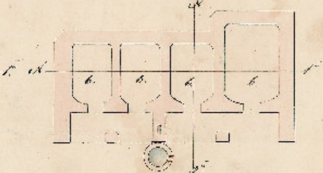
Мануфактурный котел по поверхности. план и разрез.
