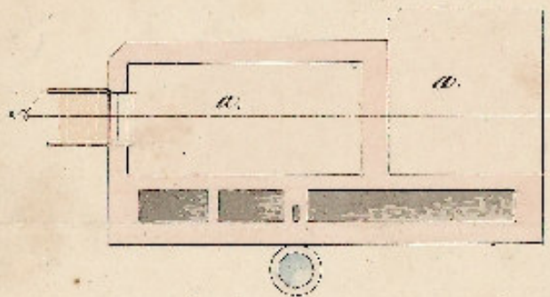
План и разрез котла.
