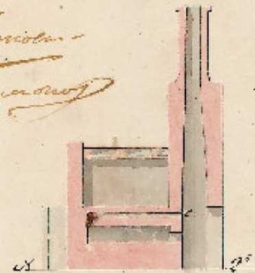
Мануфактурный котел по поверхности. план и разрез.
