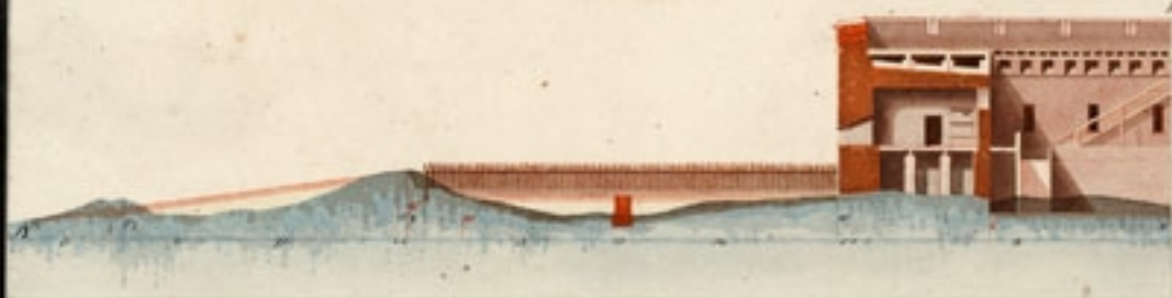
Профиль и фасадъ чрезъ левой фланг мостика первого по линіи К. 3.
